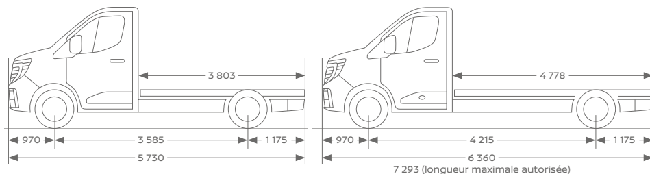
CHÂSSIS SIMPLE CABINE L2 & L3
