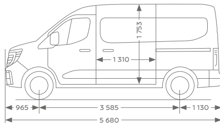
FOURGON L2 H2
