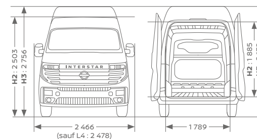
FOURGON H2 & H3
