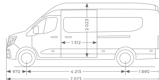
FOURGON L4 H3
