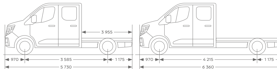
CHÂSSIS DOUBLE CABINE L3 & L4
